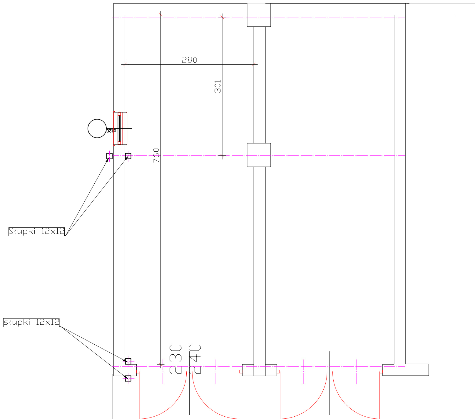
Rzut przyziemia 1:50
